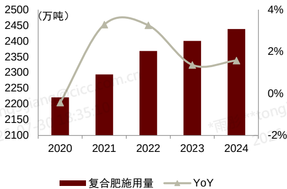
图表 39：2020-2024 国内复合肥折纯施用量 CAGR 约 2.4%
