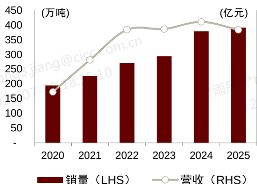
图表 8：2020-2025 年心连心尿素营业收入 CAGR 达 15%
