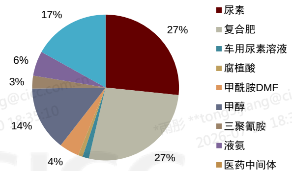
图表 5：2025 年公司营业收入结构
