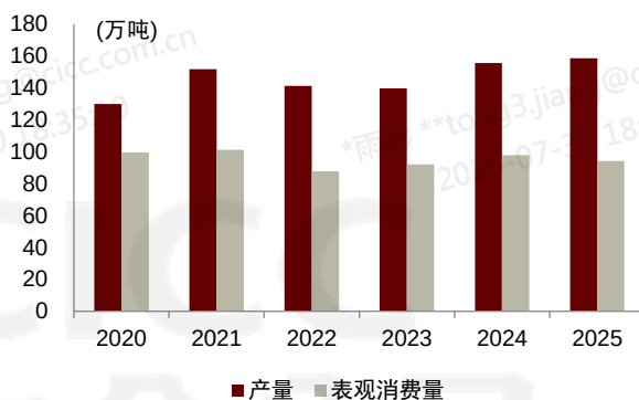
图表 23：2020-2025 年国内三聚氰胺产量 CAGR 约 4%
