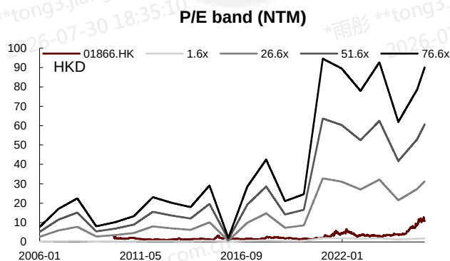
图表 54：历史 P/E
