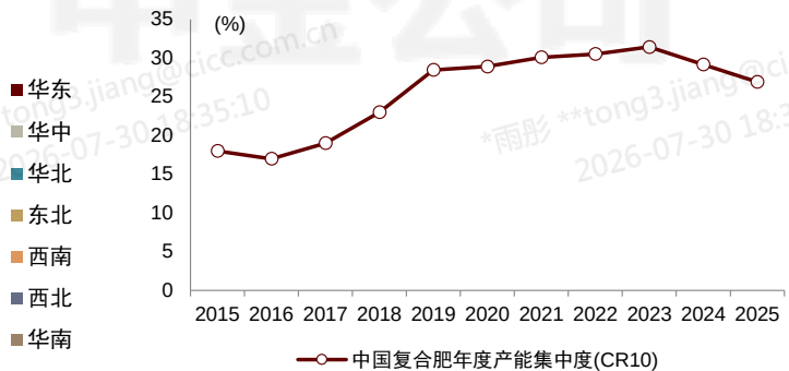
图表 36：2025 国内复合肥产能 CR10 为 27%
