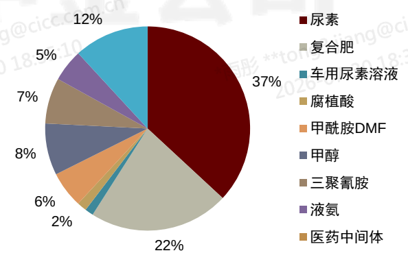
图表 7：2025 年公司毛利结构
