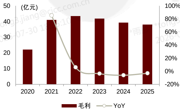
图表 6：2020-2025 年公司毛利 CAGR 达 11%
